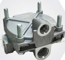
31-SORLRL3518ZA05CN รีเลย์วาล์ว BENZ, SINOTRUK (9730110010) SORL
