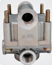
31-SORLRL3518KACN วาล์วแบ่งลมแบบสองทาง (M22x1.5) SORL
