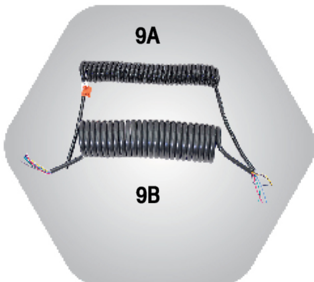
9A สายไฟคอယ် 7 สาย Phillips 636-5270 9B สายไฟคอယ် 7 สาย ขนาด 1.5 sq.mm
