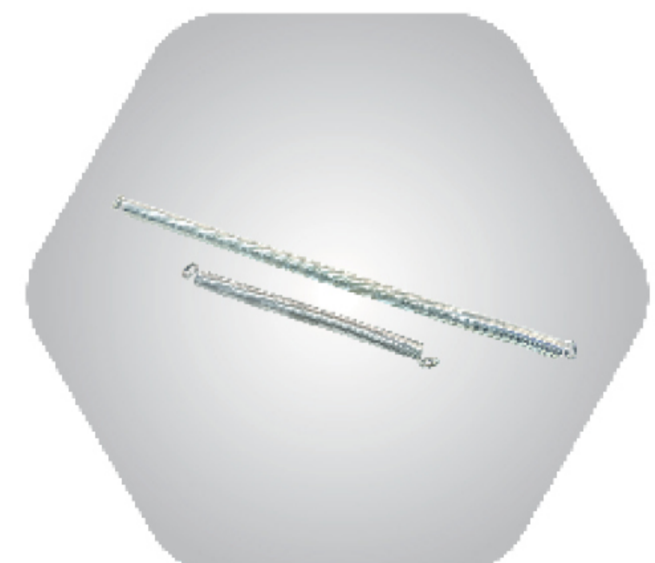
16 สปริงดึงสายลม/สายไฟ (ตัวสั้น 330 mm/ตัวยาว 620 mm)
